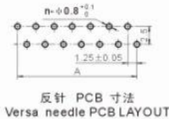
正针 PCB 寸法 Positive needle PCB LAYOUT
