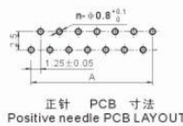
安装图 ASSEMBLY LAYOUT
