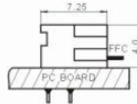
安装图 ASSEMBLY LAYOUT
